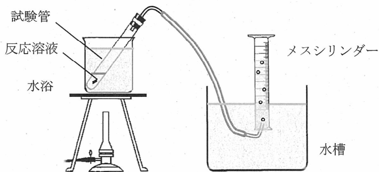
図1 実験装置
