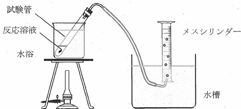
図1 実験装置
