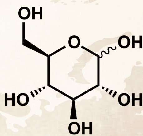
グルコース
