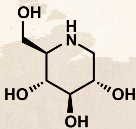
DNJ
